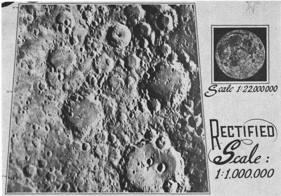
FIG. 22. Lunar mosaic, 1:1,000,000.
