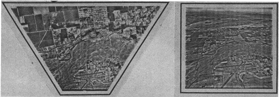
FIG. 15. 60° oblique frame rectification.
